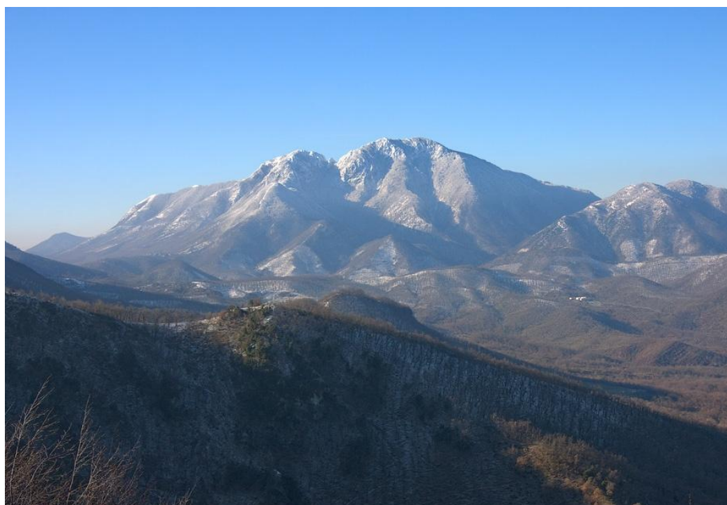
Fig. 4 Il complesso montuoso “Terminio-Cervialto”
